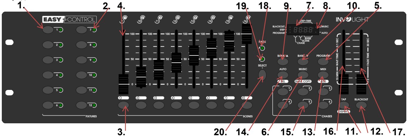
Рис. 1 Передняя панель.
